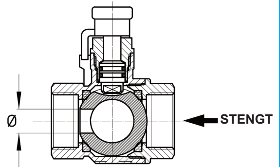
Kule med ekspansjonshull. Pilen viser ekspansjonsretning, ved stengt ventil.
