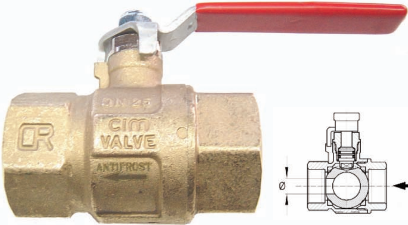
Kule med ekspansjonshull. Pilen viser ekspansjonsretning, ved stengt ventil.
